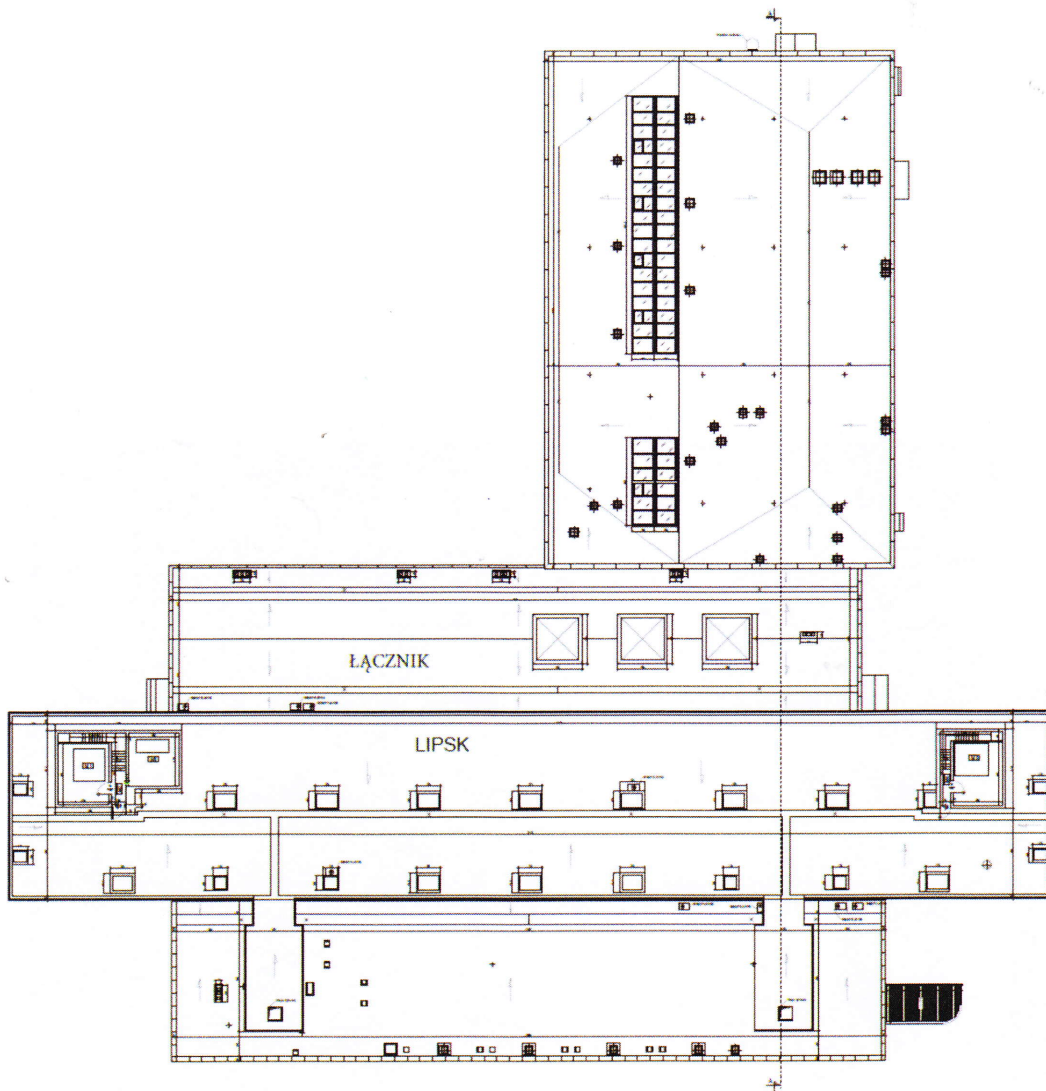
Rzut dachów
