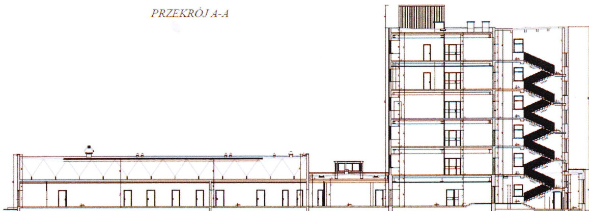
Przekrój budynków
