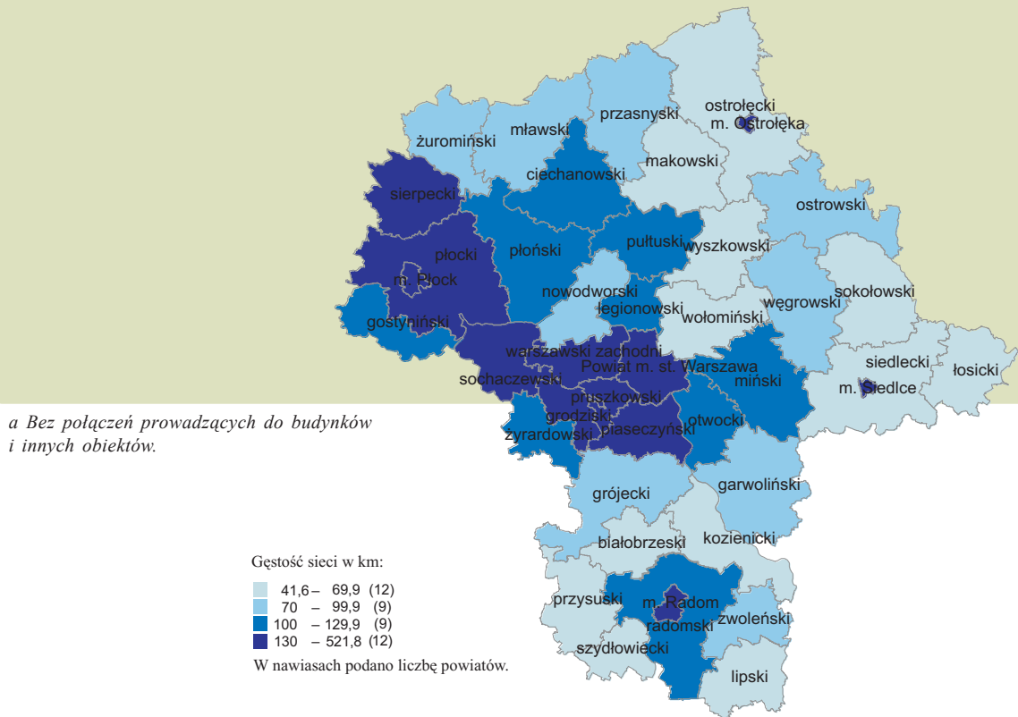
Gęstość sieci kanalizacyjnej a rozdzielczej na 100 km 2 według powiatów w 2006 r.
